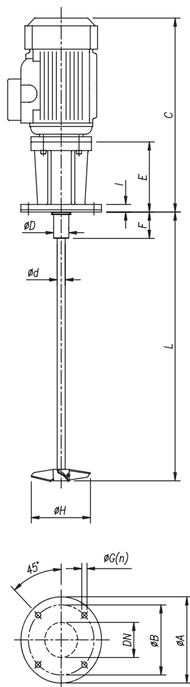
Крепление мешалки
